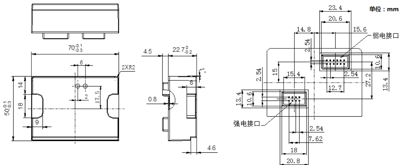
图 2 安装尺寸图
