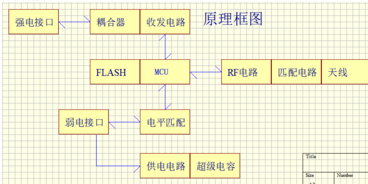
图 1 内部结构框图
